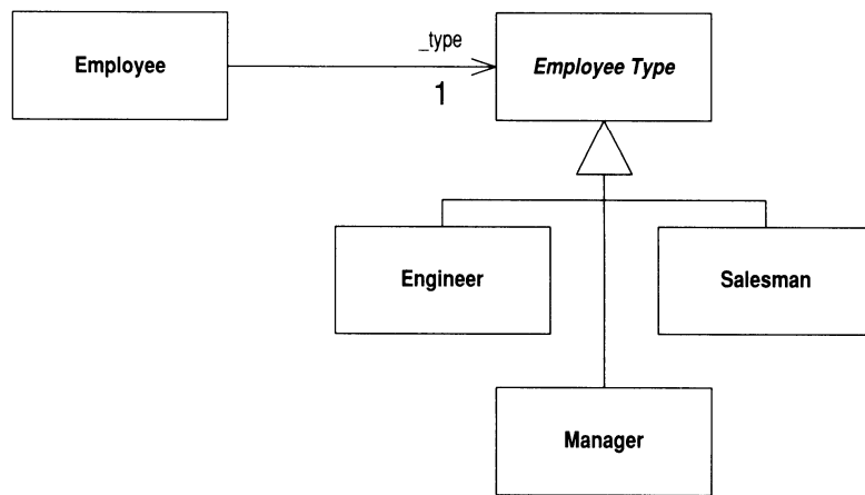
图9-1 继承结构
