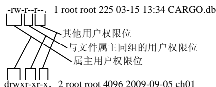
图 2-1 文件权限位示意图
