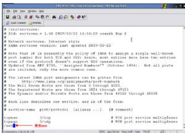
图 2-5 vi 编辑器的搜索功能
